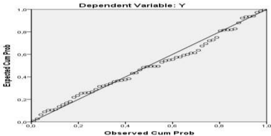
Gambar 1. Uji Normalitas
